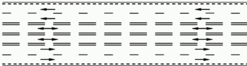
Marcaj pentru benzi cu circulația reversibilă
