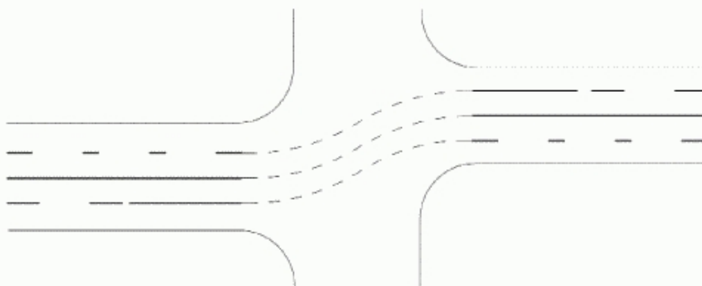
Marcaj de ghidare la traversarea unei intersecții
