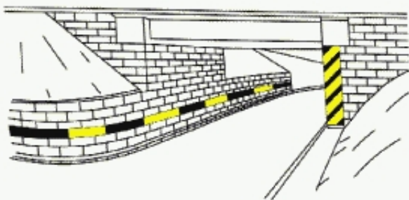
Marcaje pe ziduri de sprijin și pe infrastructurile pasajelor inferioare
