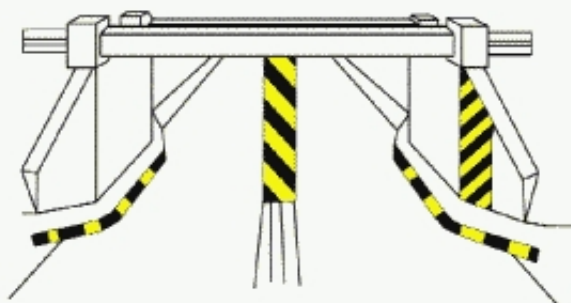
Marcaje pe ziduri de sprijin și pe infrastructurile pasajelor inferioare
